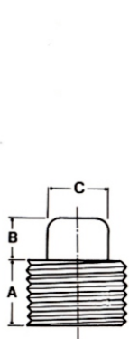
Tappi T. quadra Square H. plugs
