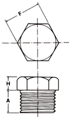
Tappi T. esag. Hex. H. plugs
