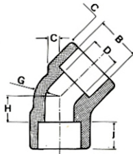
Gomiti 45° 45° Elbows
